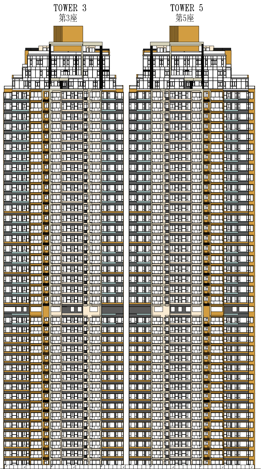
Elevation 2 立面圖 2
